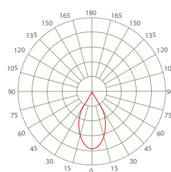
Curva fotométrica
